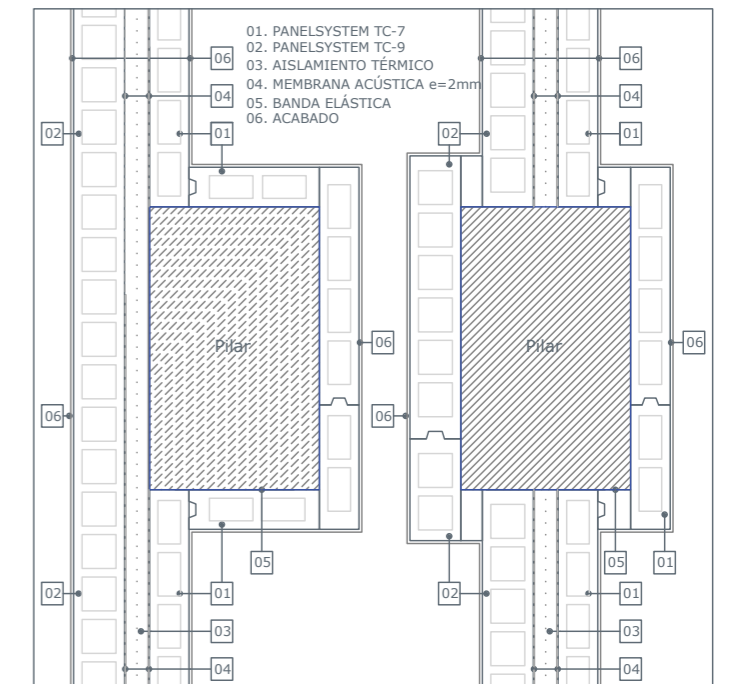
FIGURA 7b. SECCIÓN HORIZONTAL. ENCUENTRO DE UN ELEMENTO DE SEPARACIÓN VERTICAL Y UN PILAR
