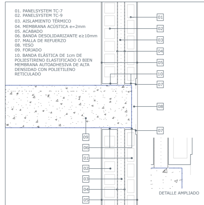
FIGURA 9a. DETALLE PARA ESCALERA
