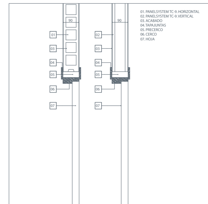
SECCIÓN VERTICAL. PARTICION INTERIOR TC-9 CON PUERTA DE PASO.
