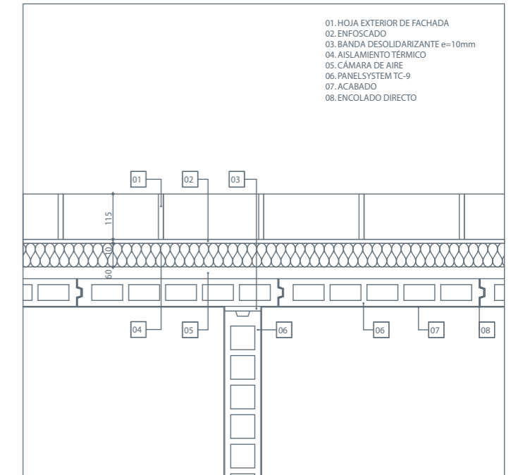
ENCUENTRO DE PARTICION INTERIOR CON TRASDOSADO. TC9
