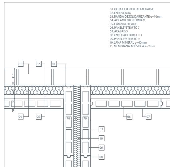
ENCUENTRO DE PARTICION INTERIOR CON FACHADA. TC7+TC9
