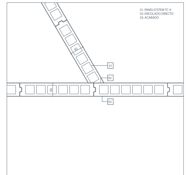
ENCUENTRO DE PARTICION INTERIOR EN ÁNGULO. TC9
