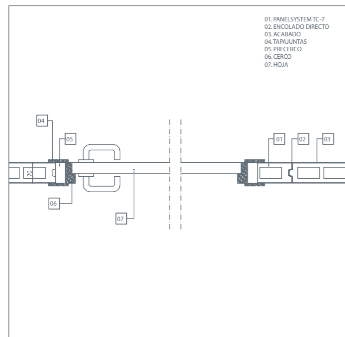
SECCIÓN HORIZONTAL. PARTICION INTERIOR TC-7 CON PUERTA DE PASO.
