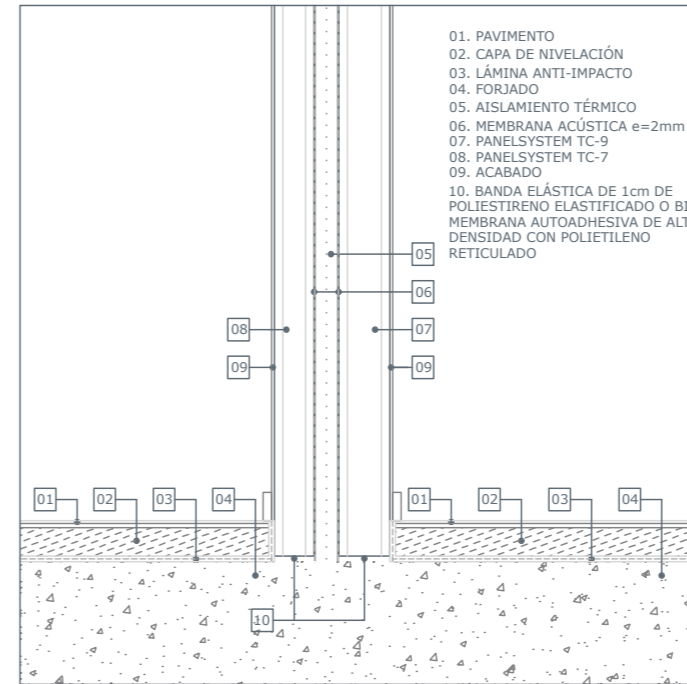
FIGURA 5a. SECCIÓN VERTICAL DE ENCUENTRO DE MEDIANERÍA CON SUELO (SOBRE FORJADO)
