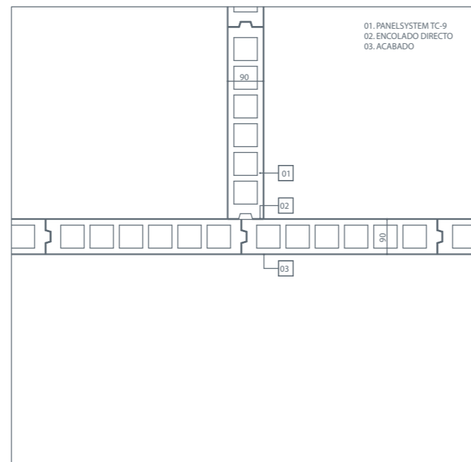
ENCUENTRO DE PARTICION INTERIOR EN T. TC9
