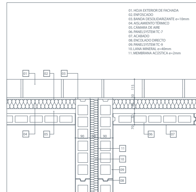
ENCUENTRO DE PARTICION INTERIOR CON FACHADA. TC9+TC9
