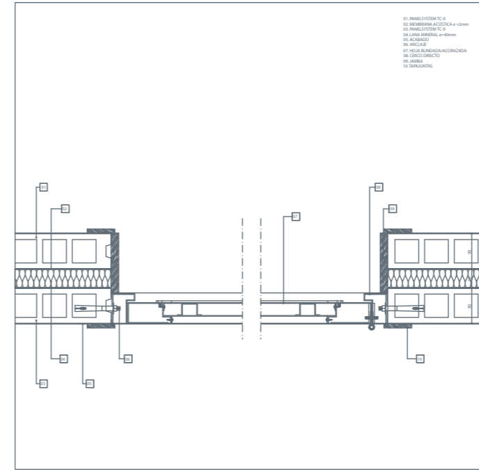
SECCIÓN HORIZONTAL. MEDIANERÍA TC-9+TC-9 CON PUERTA DE ENTRADA
