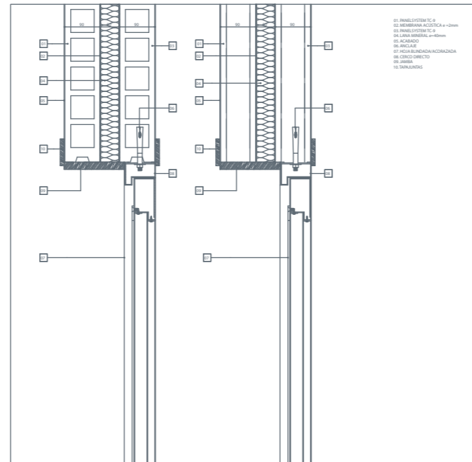
SECCIÓN VERTICAL. MEDIANERÍA TC-9+TC-9 CON PUERTA DE ENTRADA
