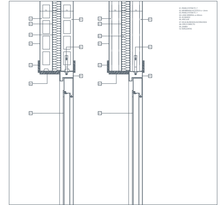
SECCIÓN VERTICAL. MEDIANERÍA TC-7+TC-7 CON PUERTA DE ENTRADA
