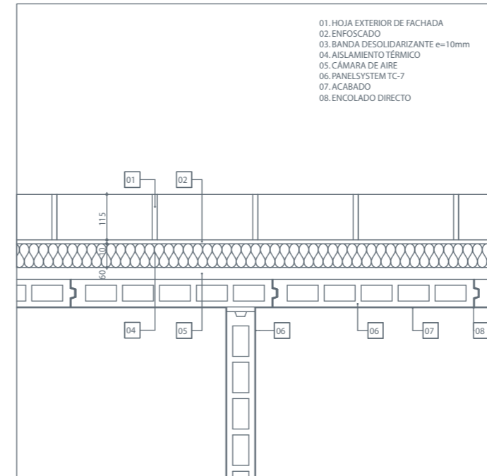
ENCUENTRO DE PARTICION INTERIOR CON TRASDOSADO. TC7
