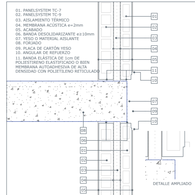
FIGURA 9b. DETALLE PARA ESCALERA
