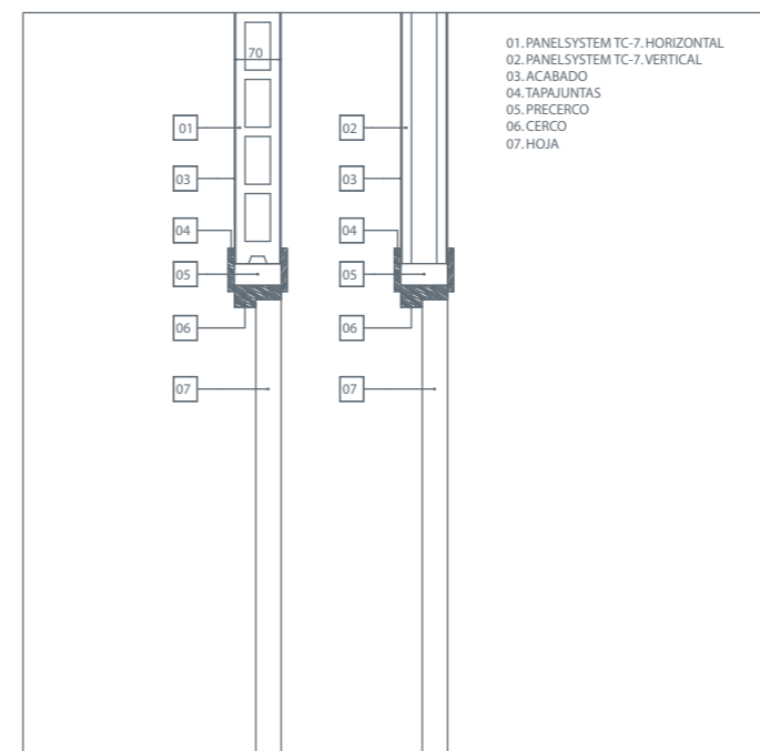
SECCIÓN VERTICAL. PARTICION INTERIOR TC-7 CON PUERTA DE PASO.
