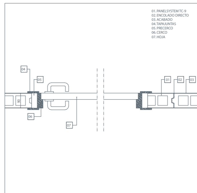
SECCIÓN HORIZONTAL. PARTICION INTERIOR TC-9 CON PUERTA DE PASO.
