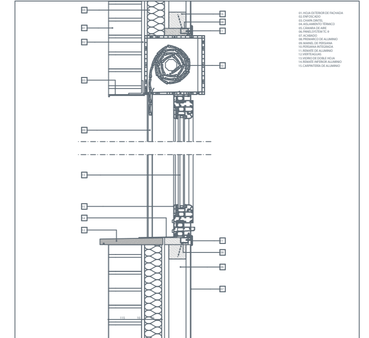
SECCIÓN VERTICAL POR VENTANA DE CARPINTERÍA DE ALUMINIO. TRASDOSADO TC9
