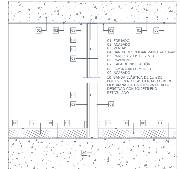
FIGURA 5b. SECCIÓN VERTICAL DE ENCUENTRO DE PANEL CON SUELO (SOBRE FORJADO)
